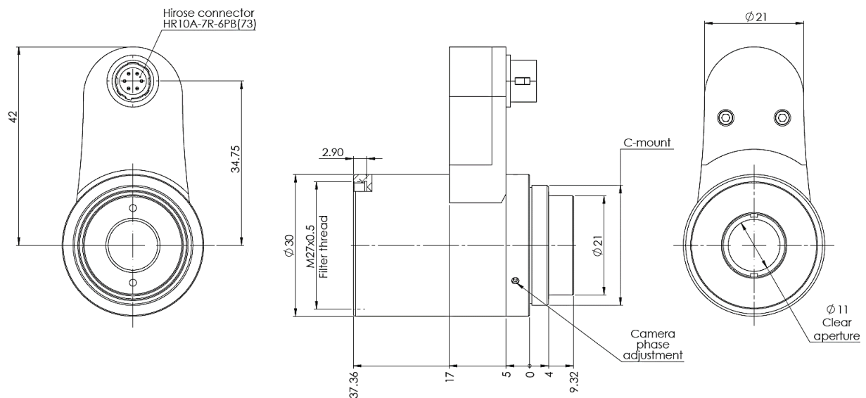
图 1: ELM-12-5.6-11-C 的机械图纸
