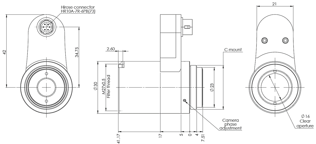
图 1: ELM-16-5.6-11-C 机械图纸
